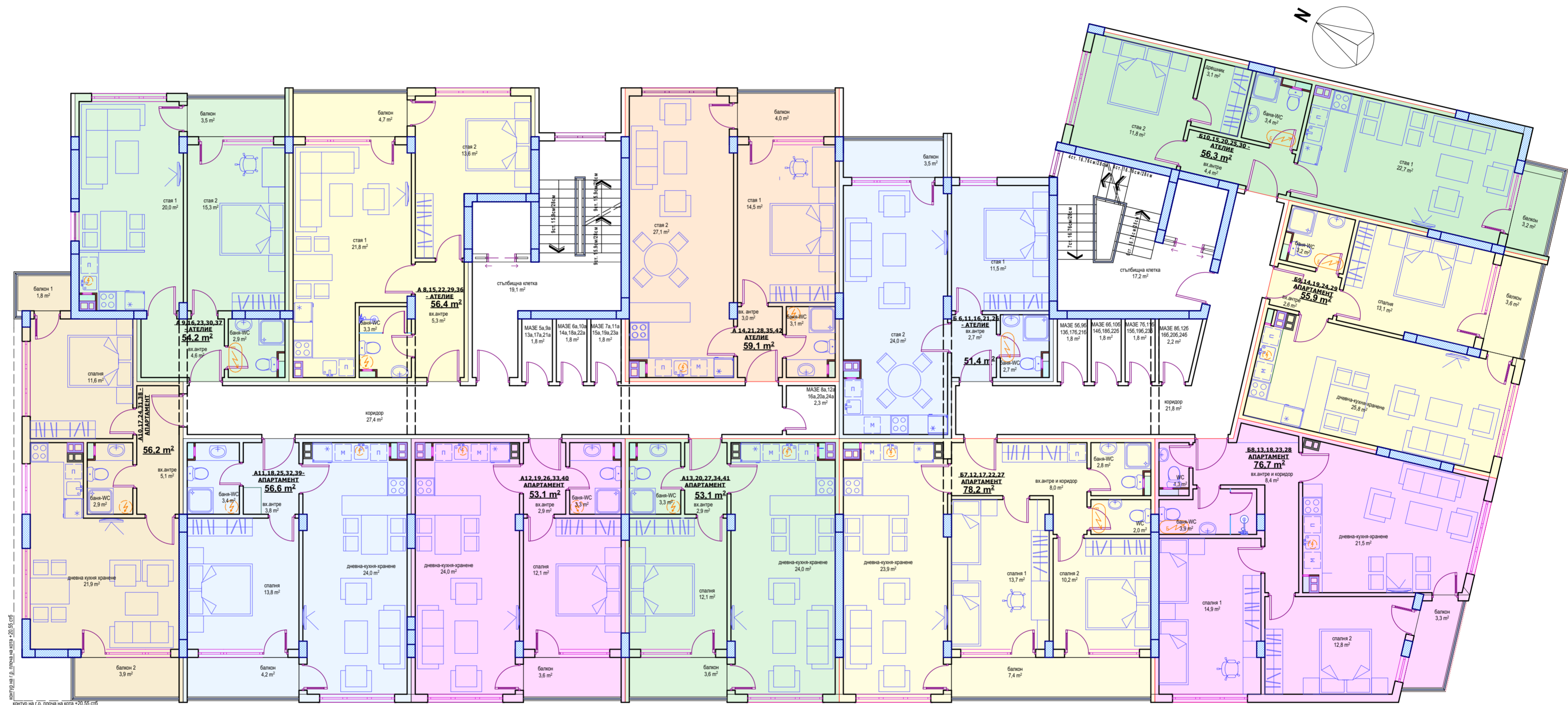
ПЛАН РАЗПРЕДЕЛЕНИЕ ТИПОВ ЕТАЖ НА КОТА +6.35 , 9.20 , 12.05 , 14.90 , 17.75
