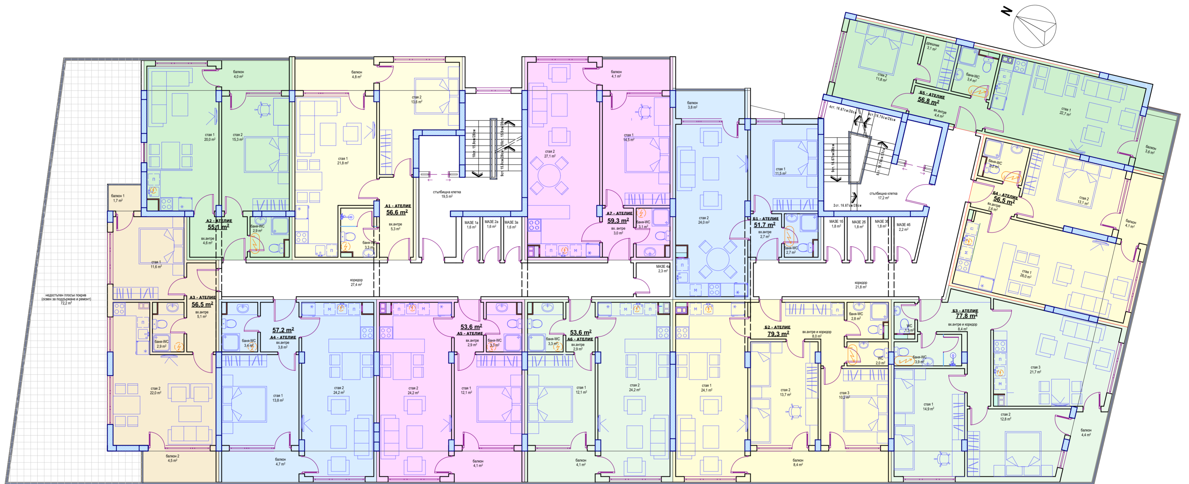
ПЛАН РАЗПРЕДЕЛЕНИЕ НА КОТА +3.50
